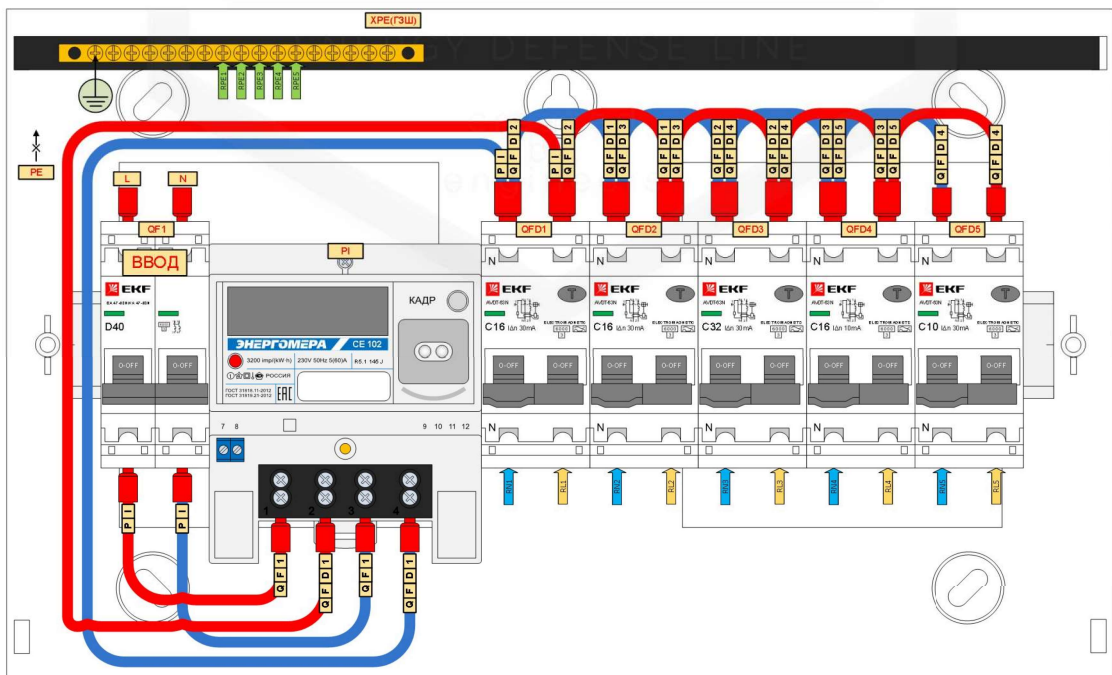
Подключение к системам TN-S и TN-C-S с переформированием в TT
