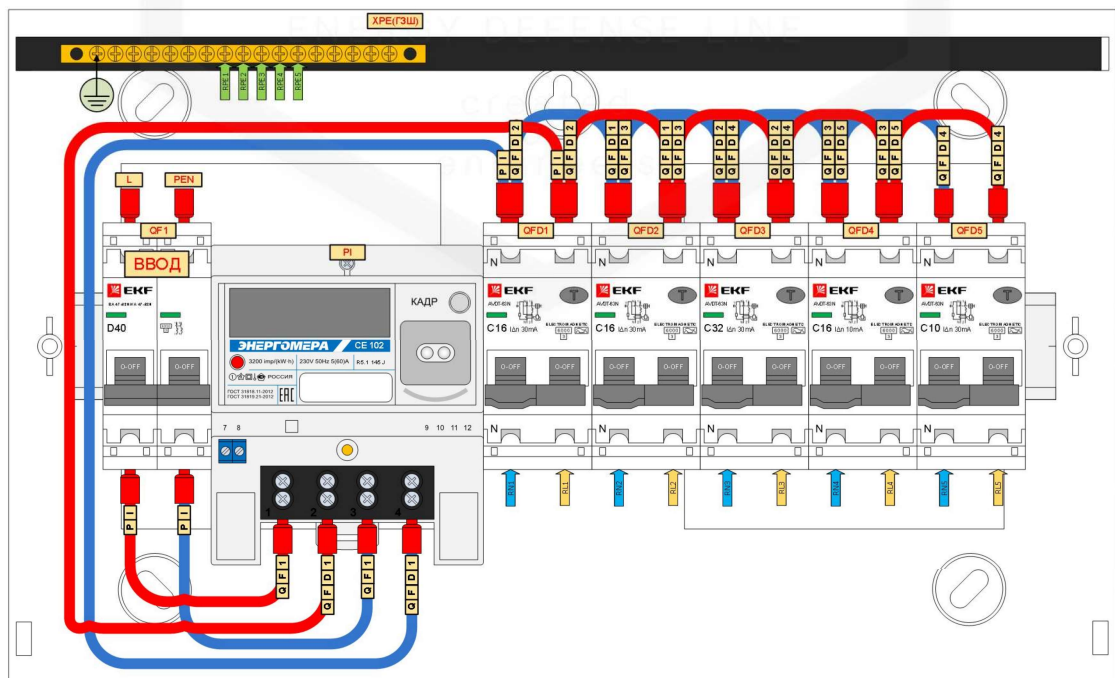
Подключение к системе TN-C с переформированием в TT
