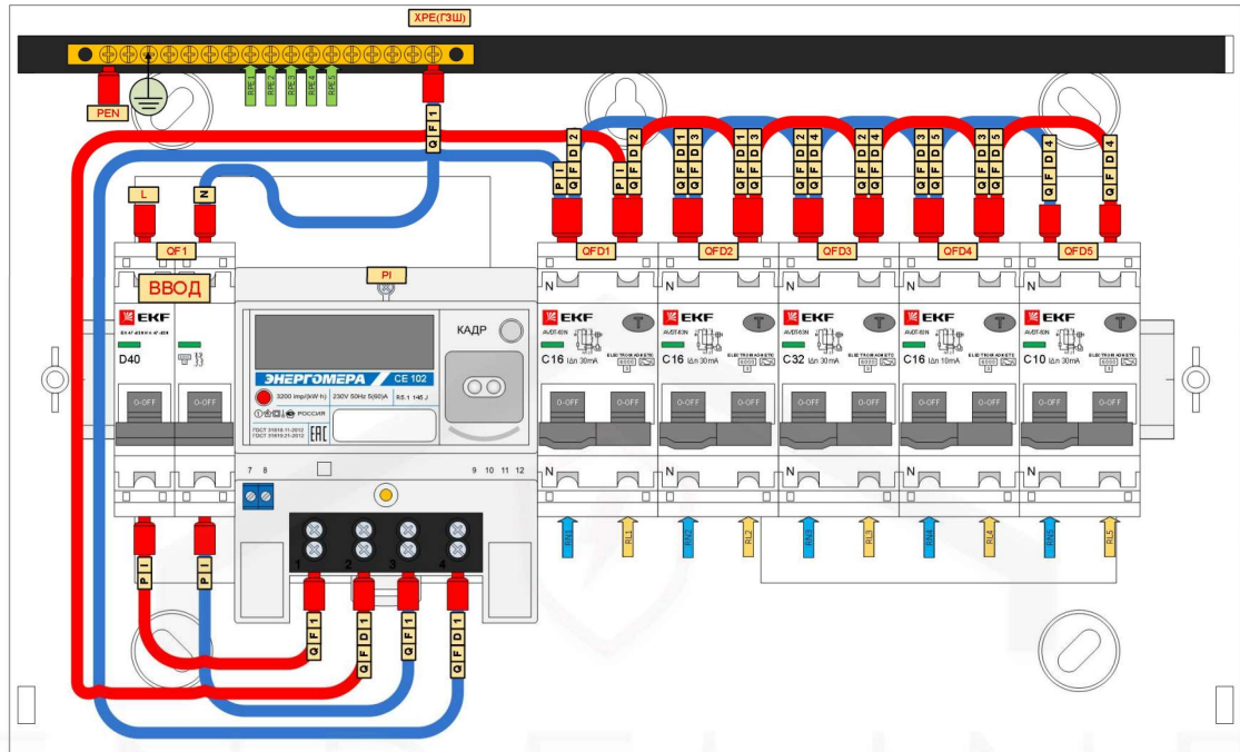
Подключение к системе TN-C с переформированием в TN-C-S
